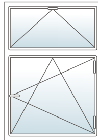
Draaikip rechts met valraam
