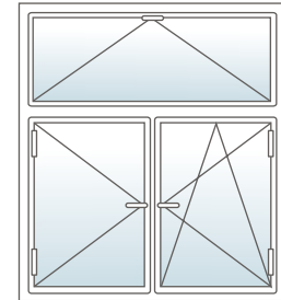
Dubbeldraaikip rechts met valraam
