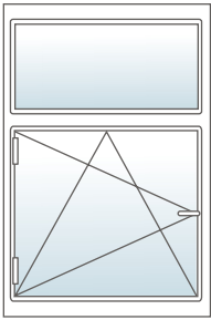
Draaikip links met bovenlicht
